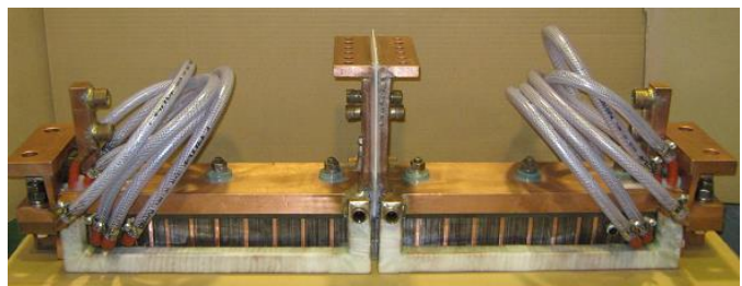
端面加熱コイル
