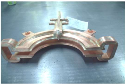
ディスクプレート加熱コイル
